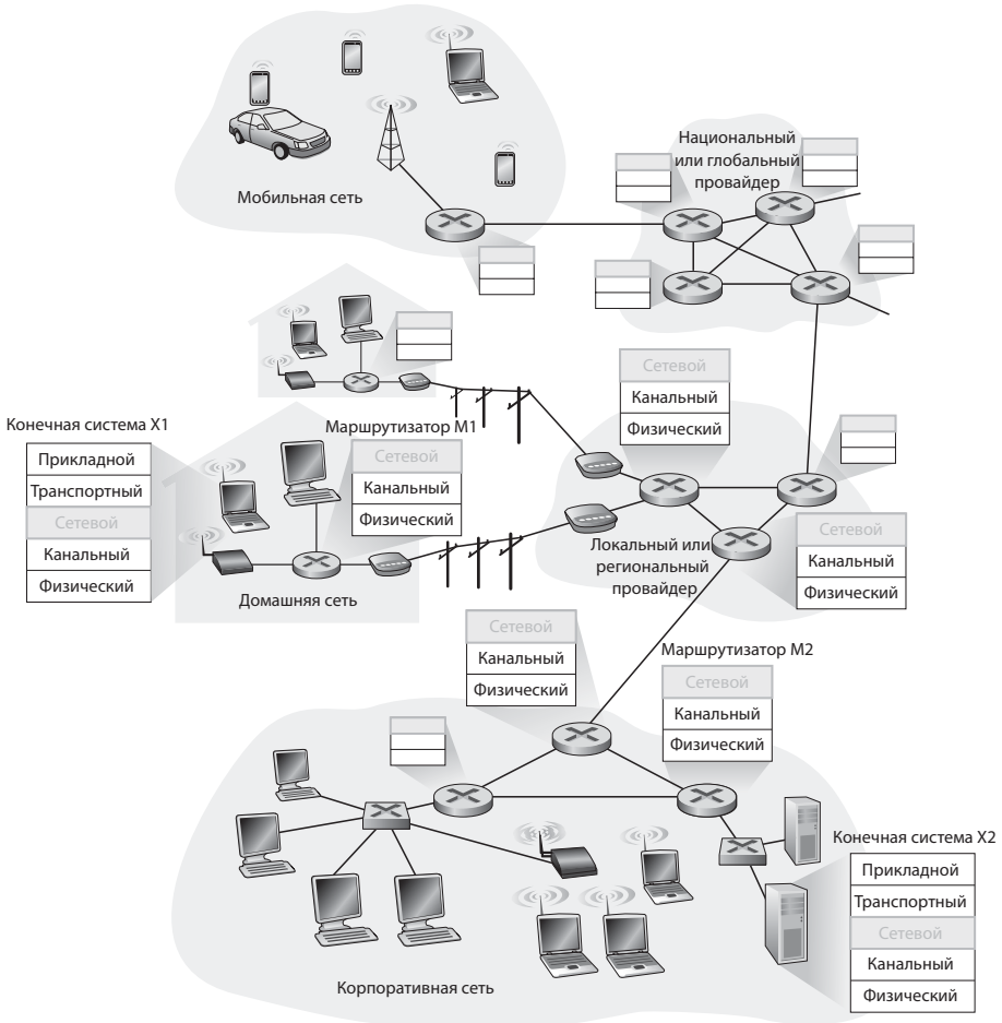
Рис. 4.1. Сетевой уровень
