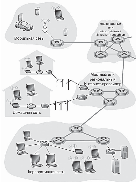
Рис. 1.10. Ядро сети
