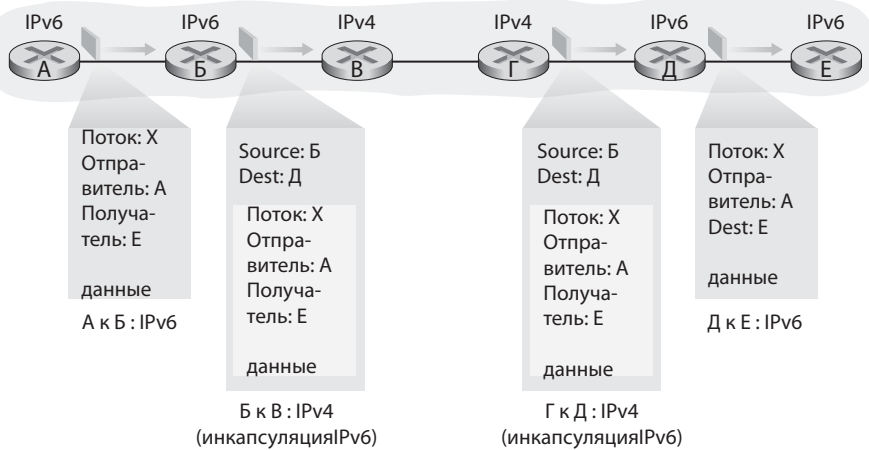
Рис. 4.26. Туннелирование
