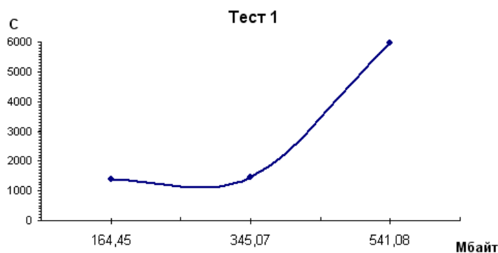
Рис. 2: Тесты утилит ngindex и ngfilter
