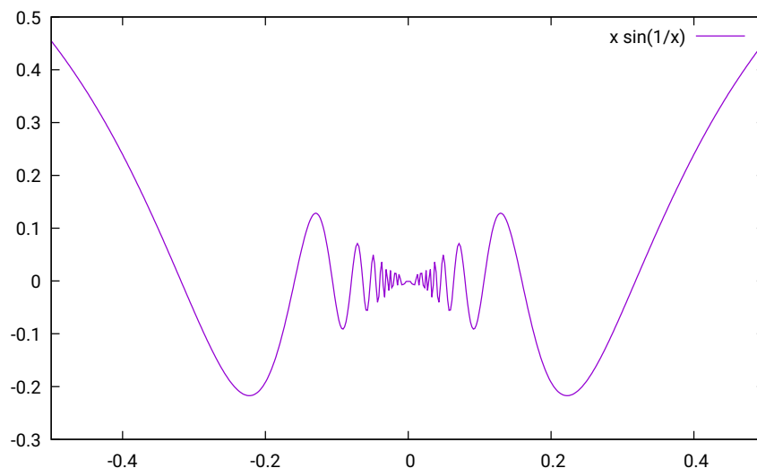
Рис. 1: График функции x \sin(\frac{1}{x})
