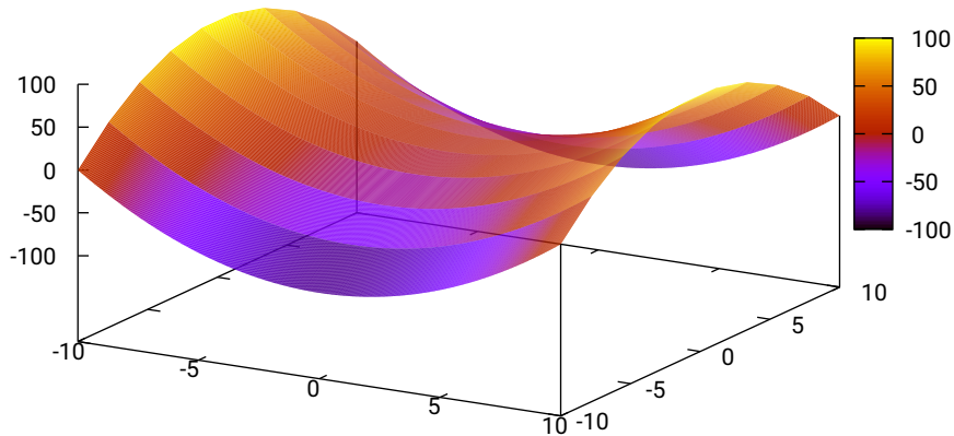
Гиперболический Параболоид
