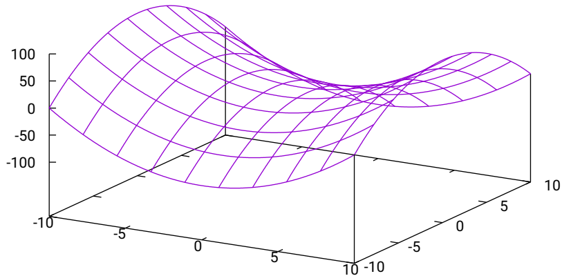
Гиперболический Параболоид —
