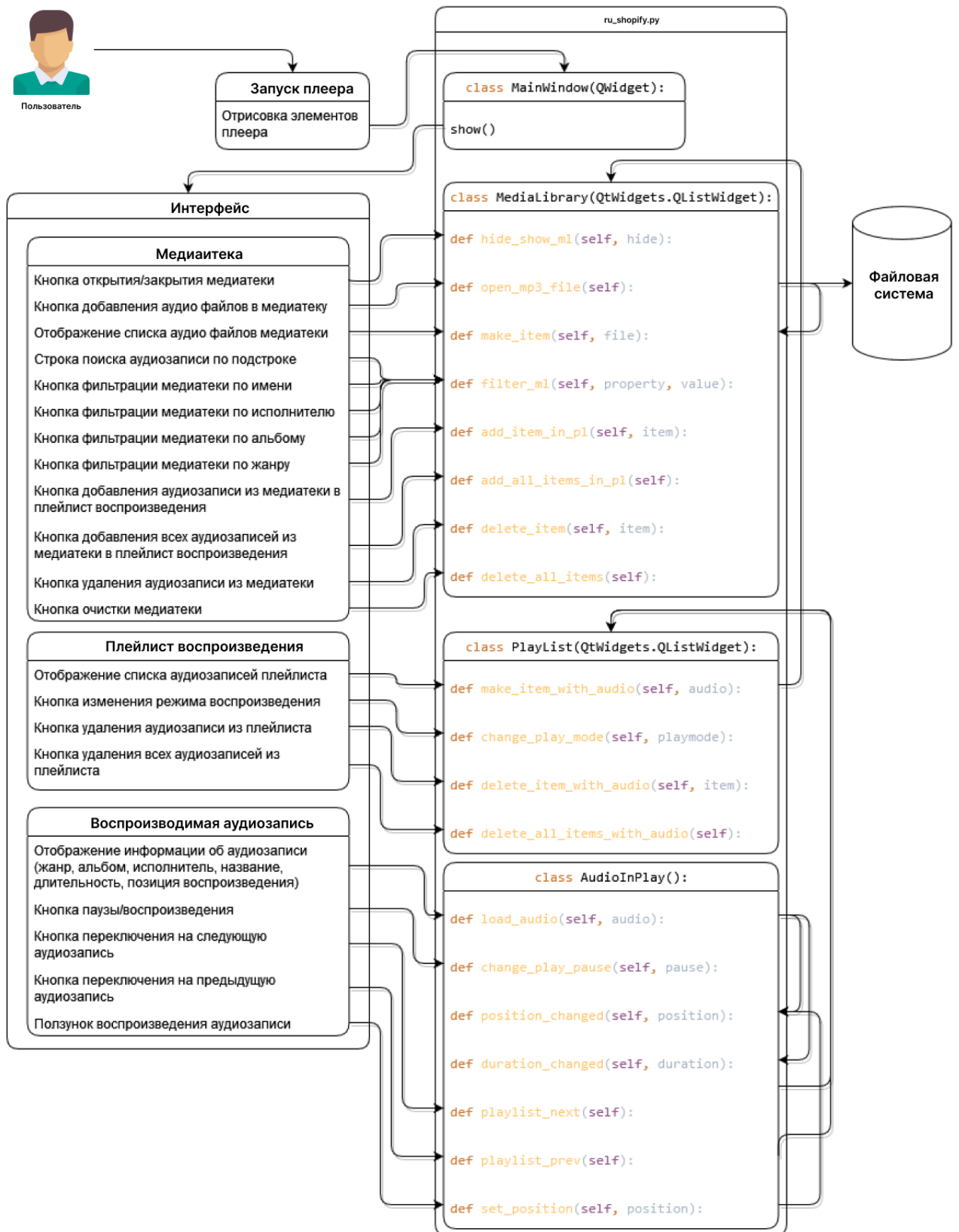
Рис. 2: Архитектура приложения
