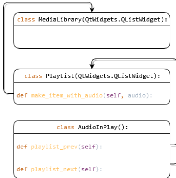
Рис. 1: Связи модулей
